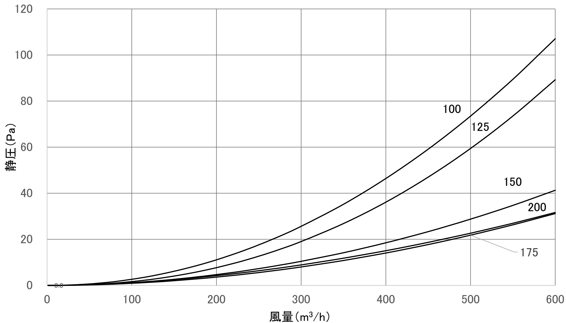
風量特性曲線 SKEA(排気)
