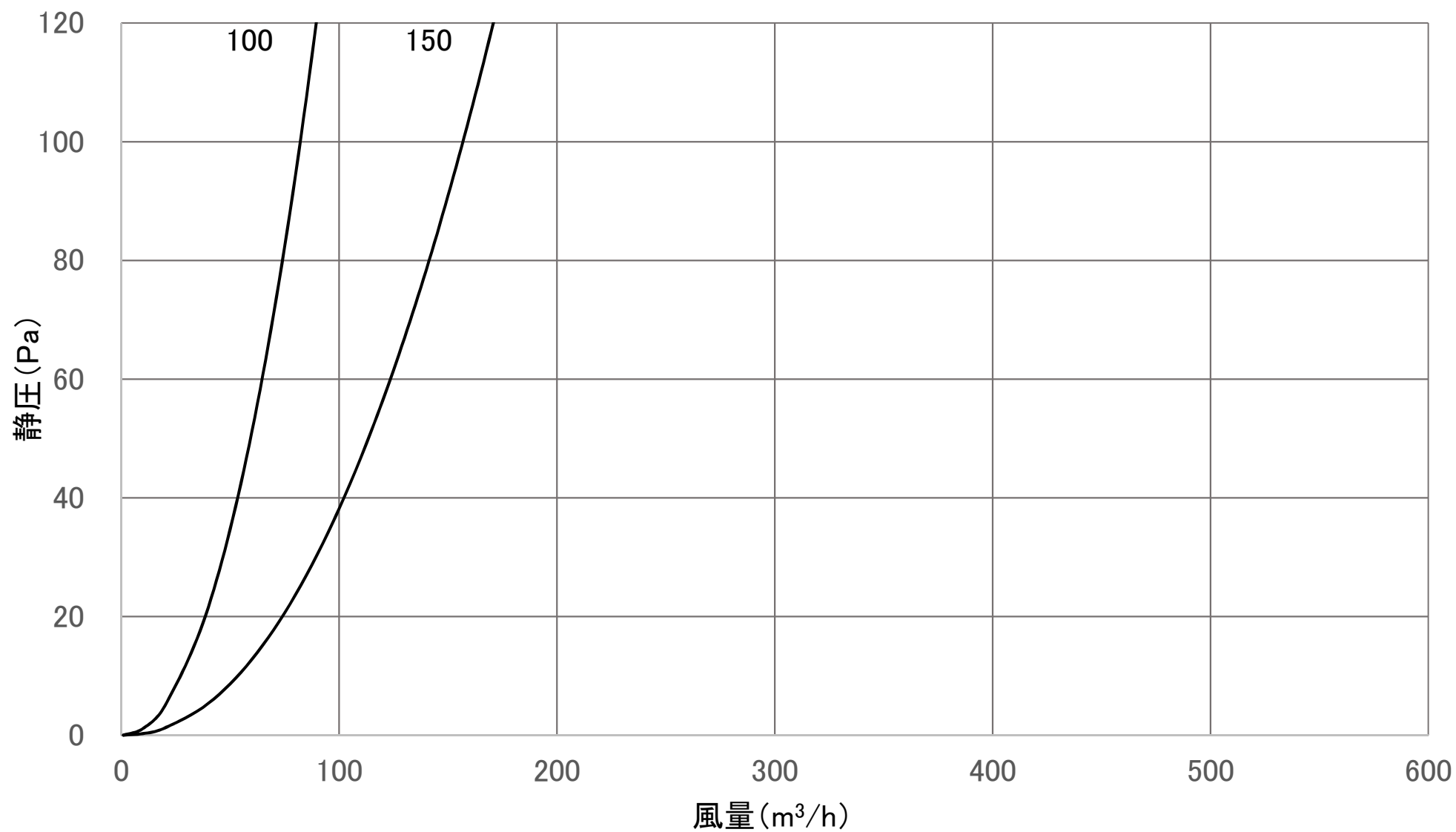
風量特性曲線 SFOA-10M(吸気)
