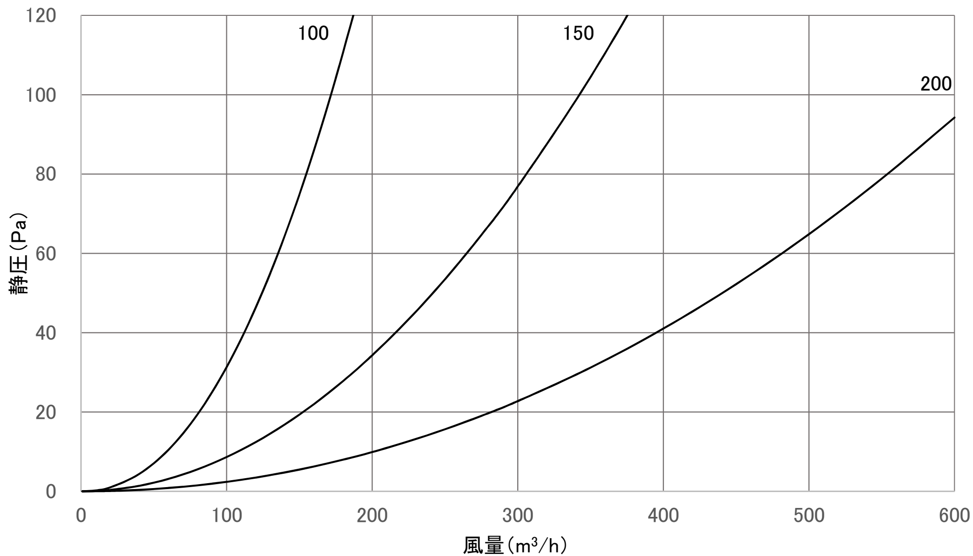
風量特性曲線 SFG2(排気)
