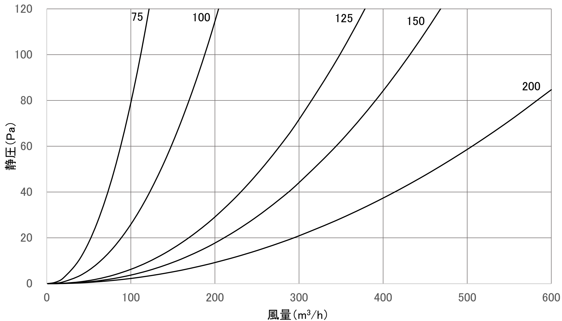
風量特性曲線 RHG-D(排気)
