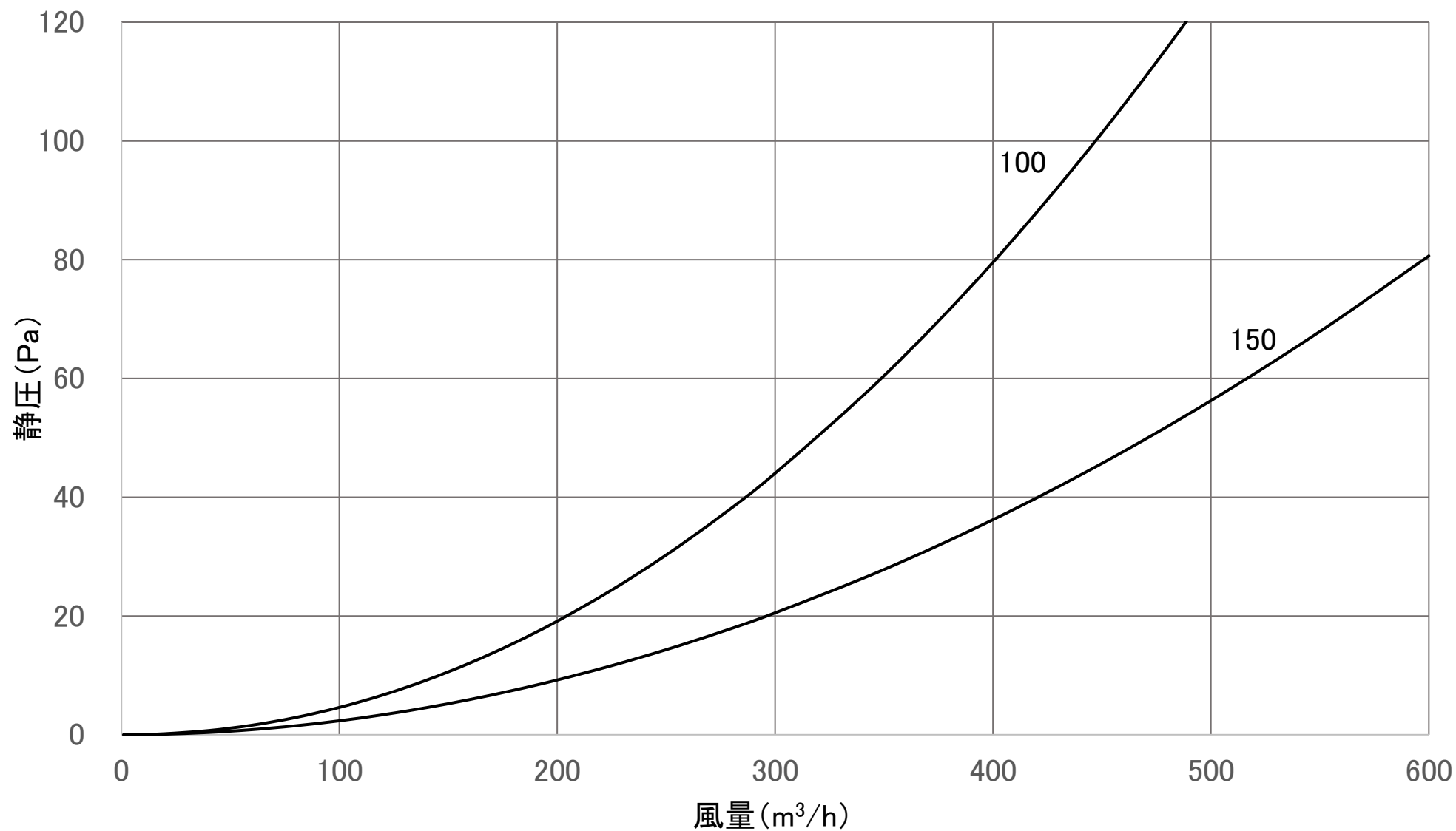
風量特性曲線 CSGB(排気)
