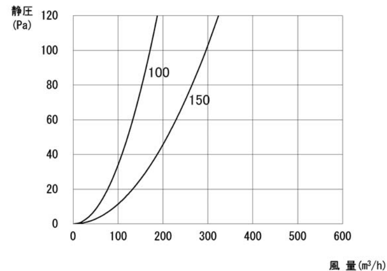
圧力損失曲線
