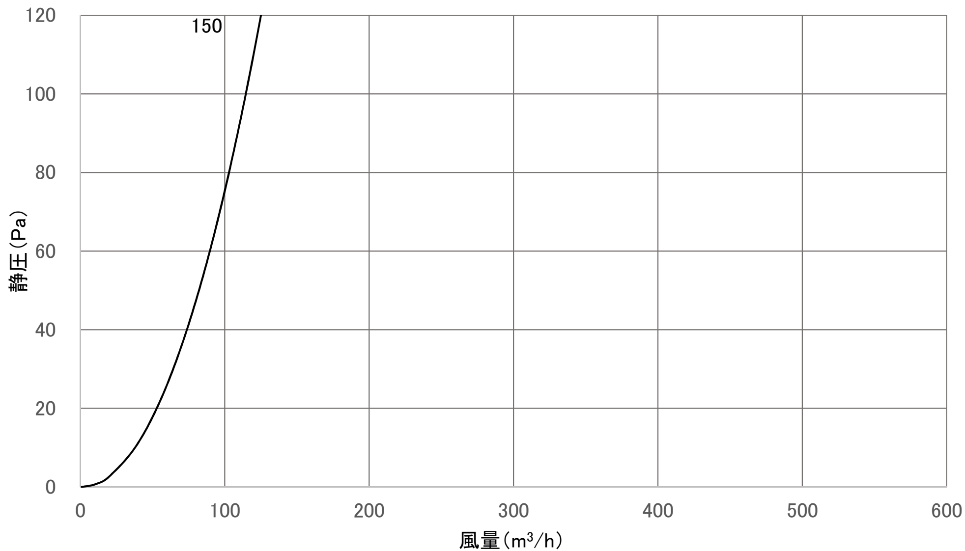
風量特性曲線 BONTT-10M(吸気)
