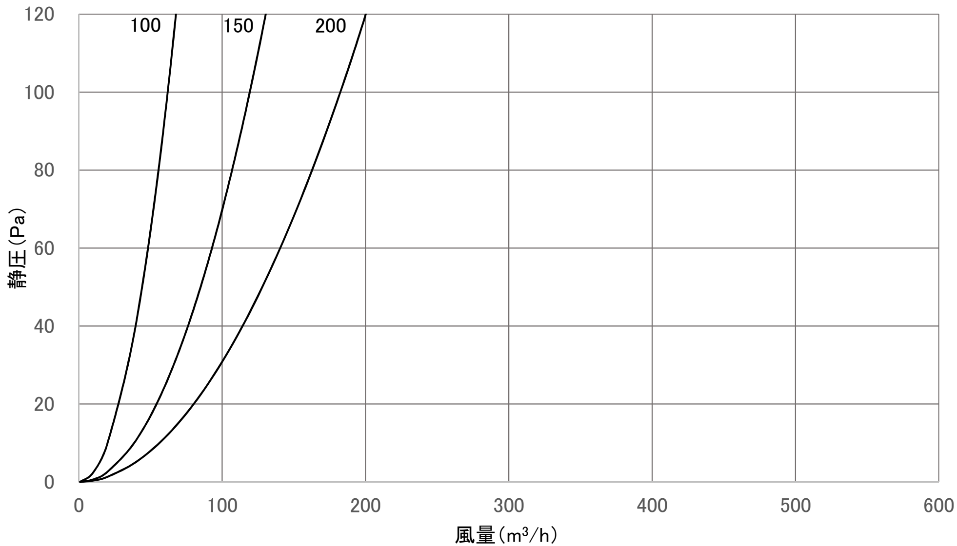
風量特性曲線 BONT-10M(吸気)
