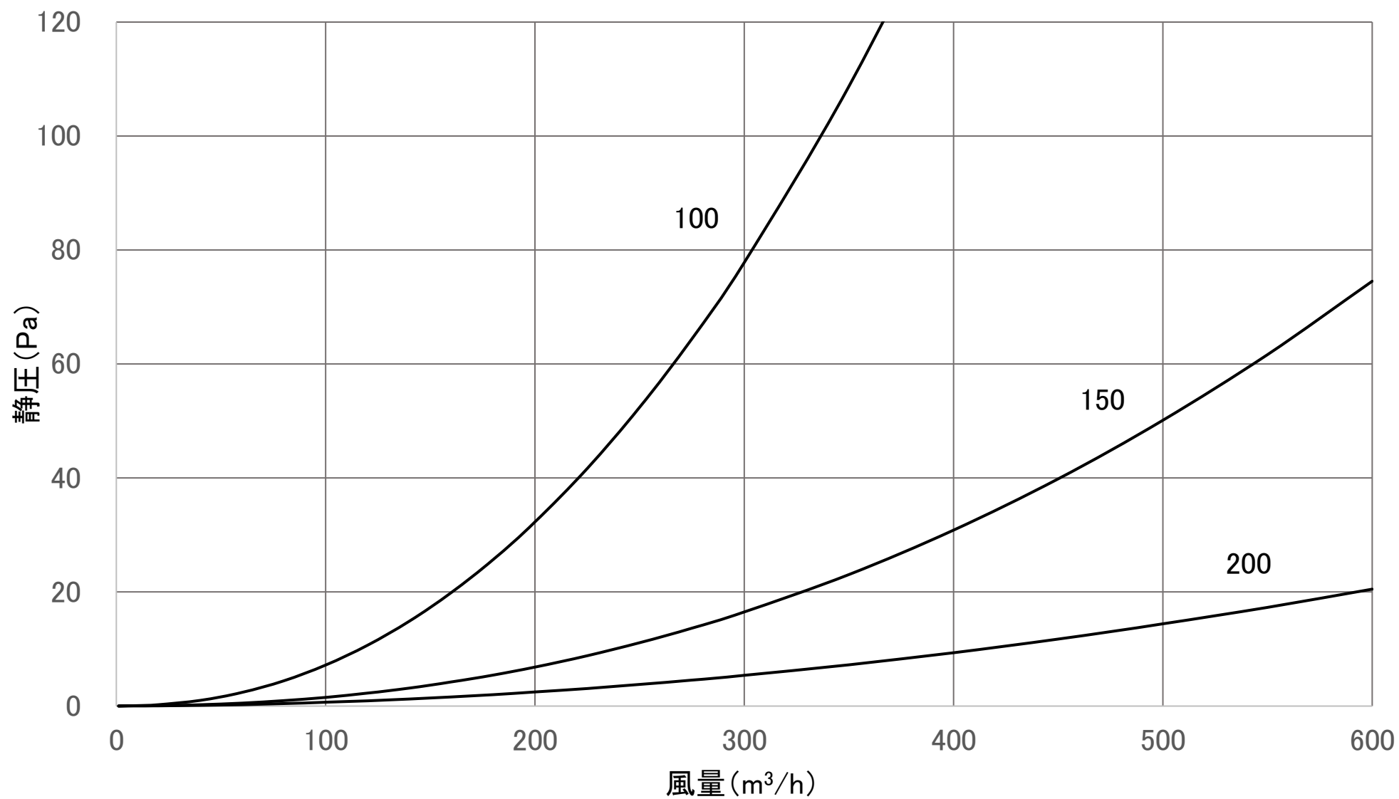
風量特性曲線 CSG2(排気)
