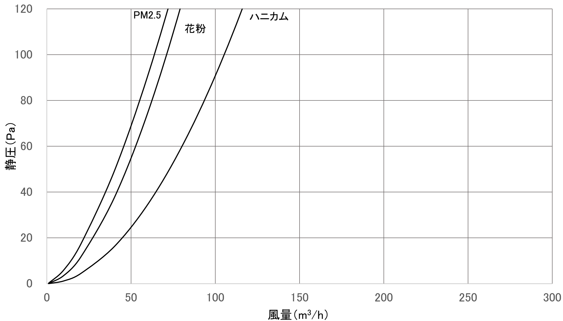
風量特性曲線 PITS2-100(全開)
