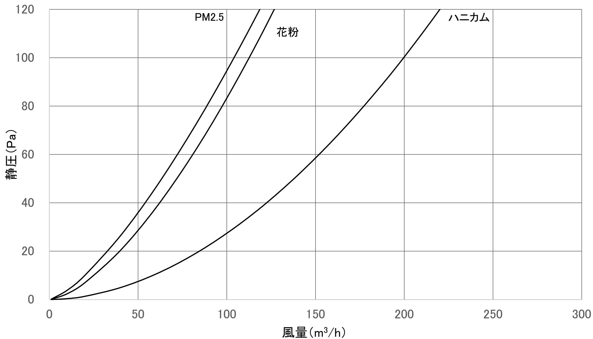
風量特性曲線 PITS2-150(全開)
