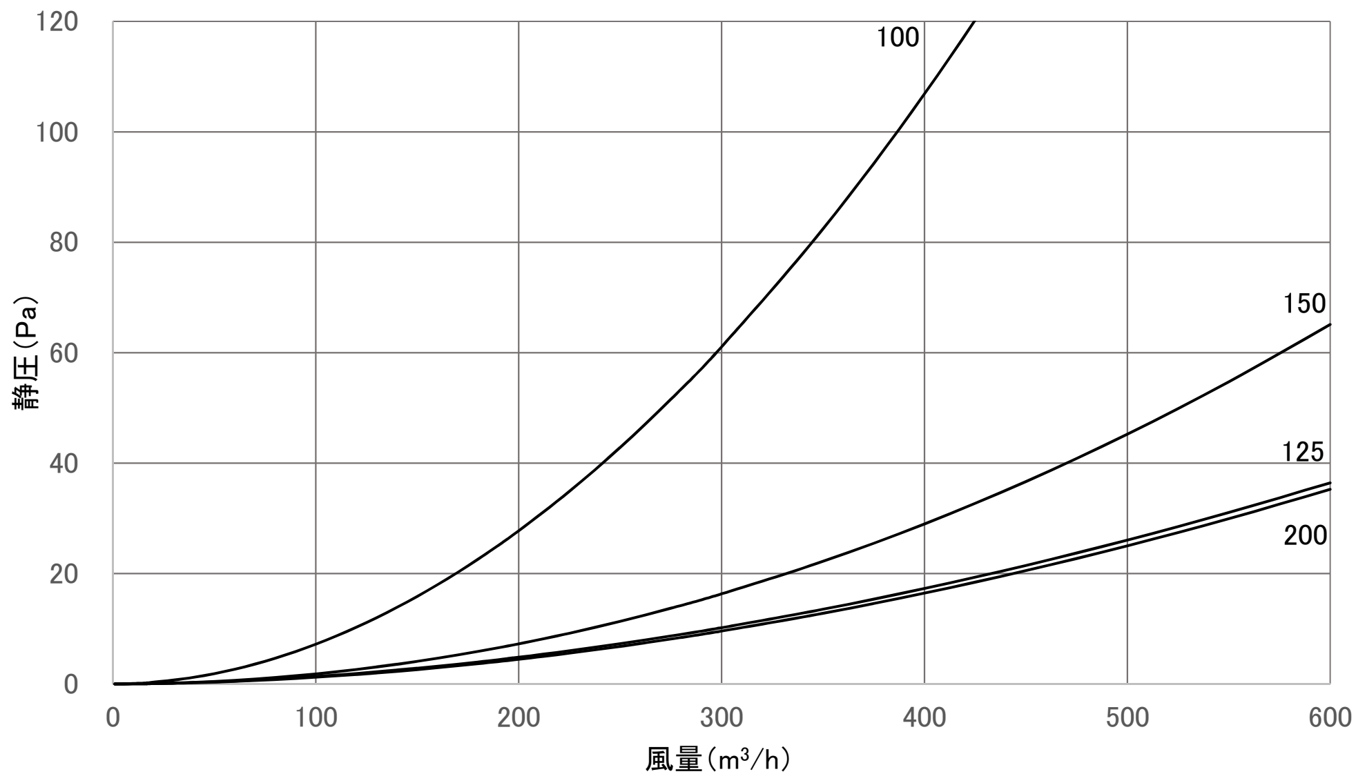
風量特性曲線 OHS(排気)
