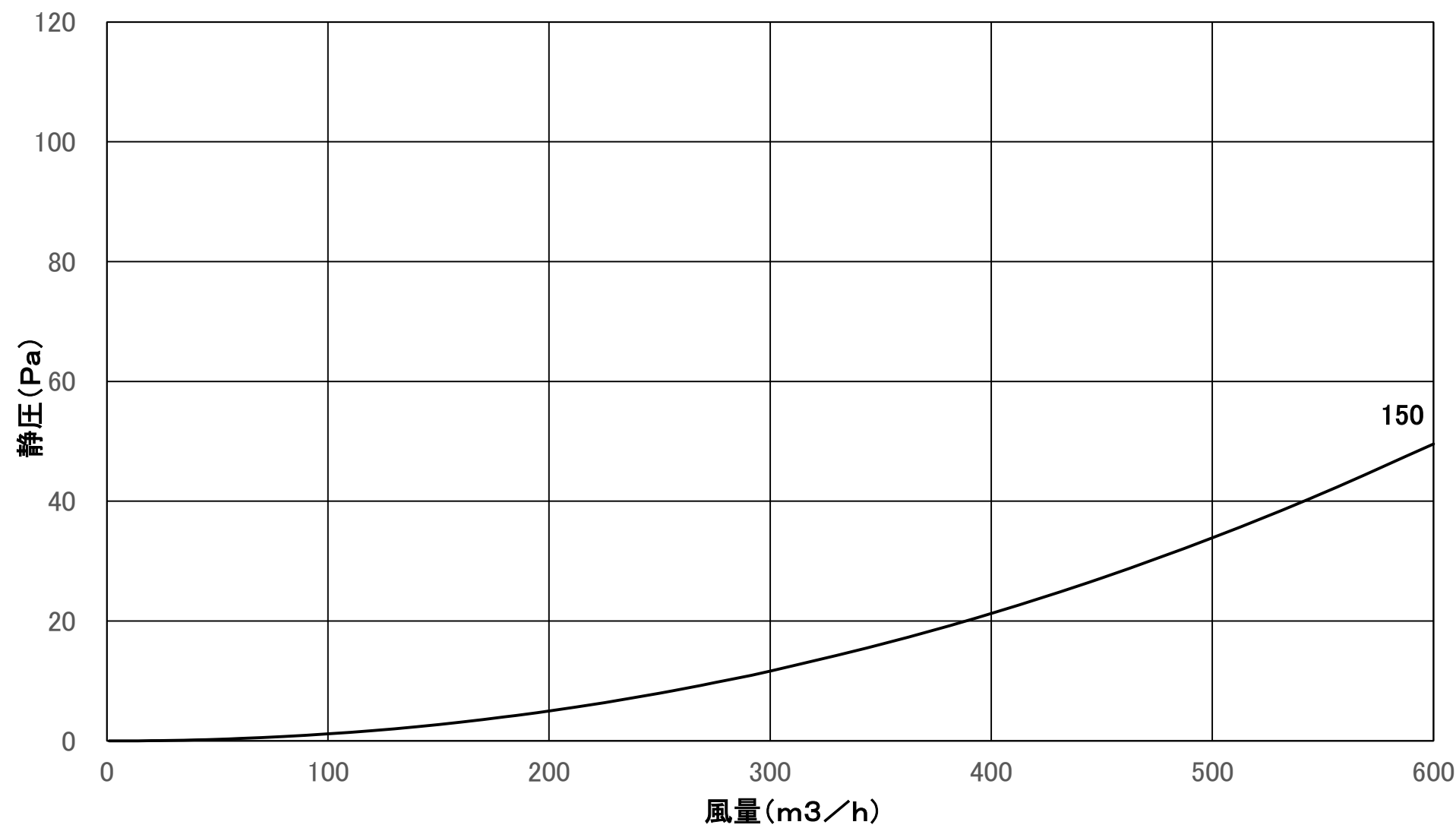
風量特性曲線 3KO-150D（排気）
