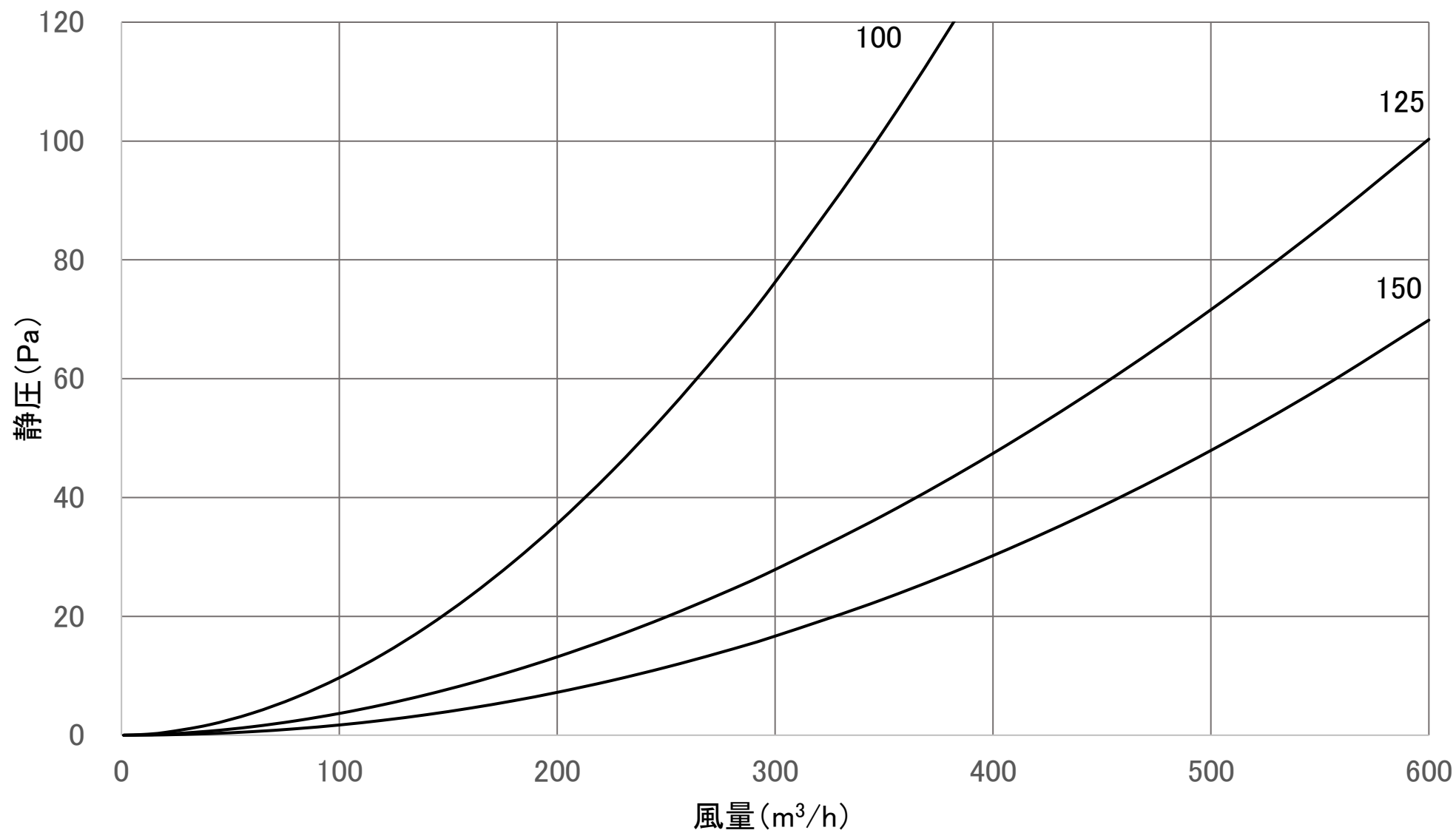
風量特性曲線 WB(排気)
