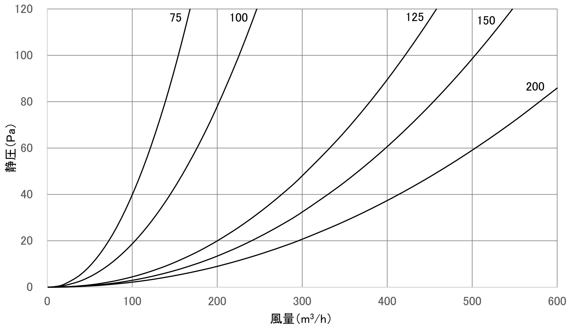
風量特性曲線 RHG(排気)
