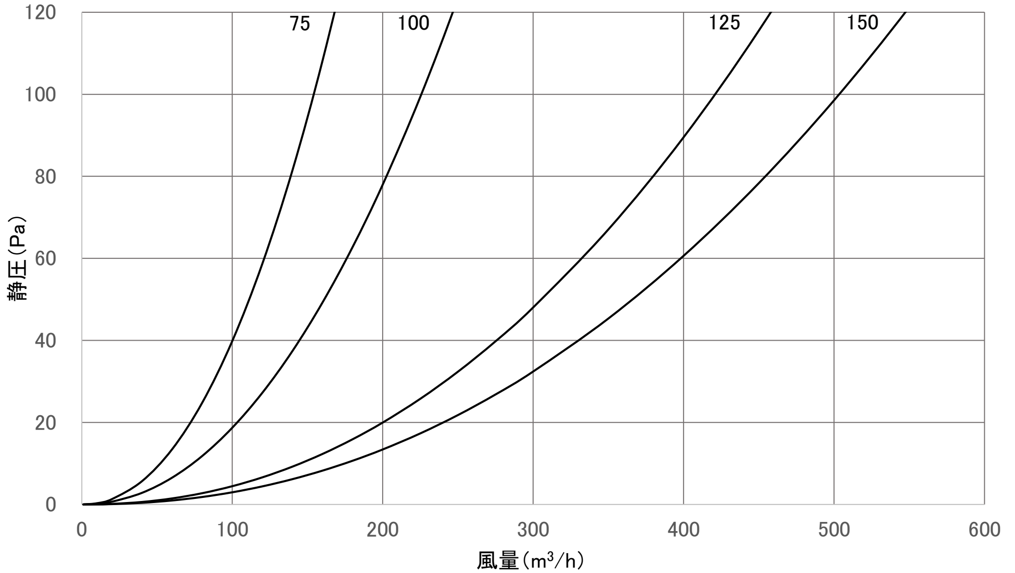
風量特性曲線 RH-YGE2(排氣)
