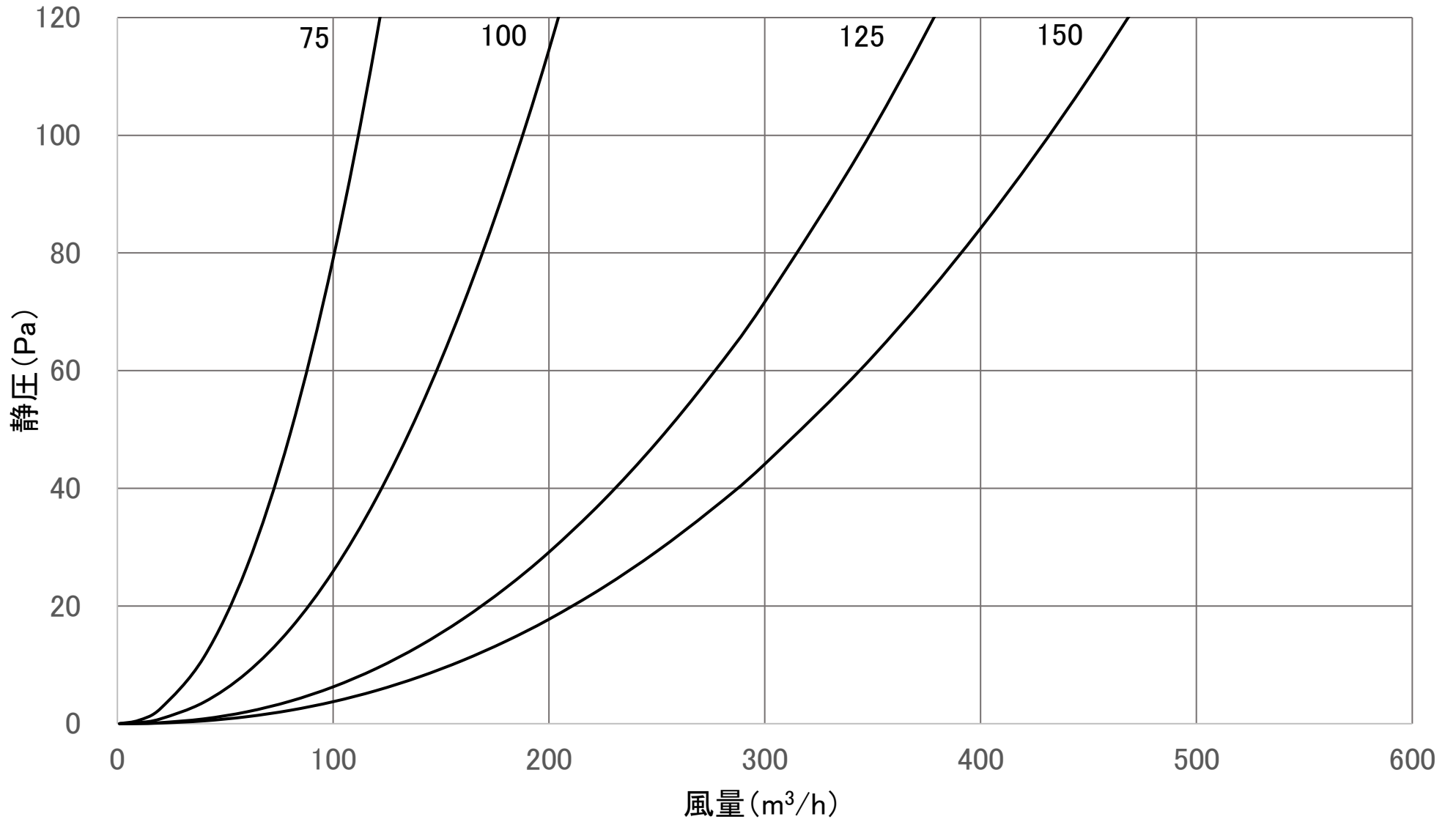
風量特性曲線 RH-YGDE2(排氣)
