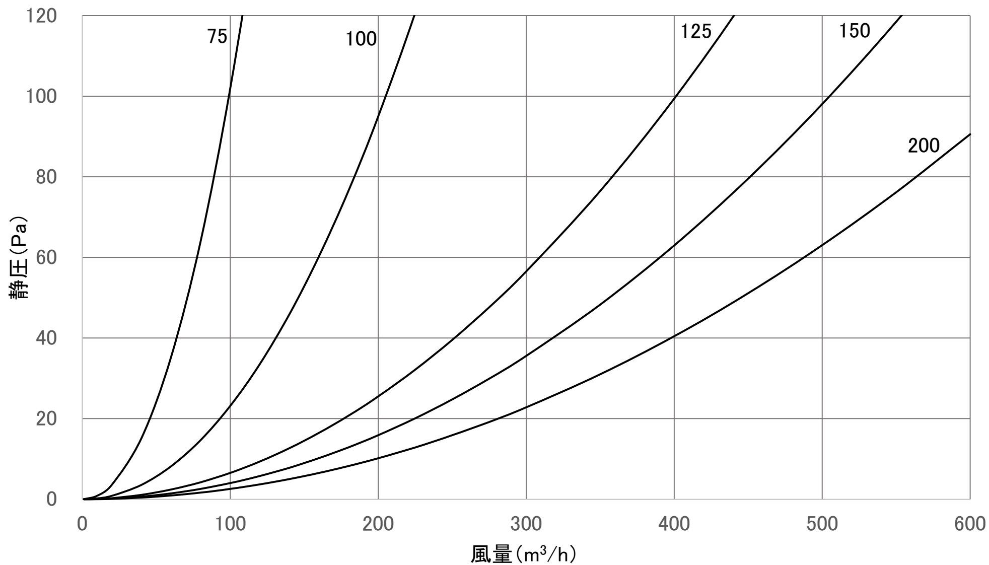
風量特性曲線 RH-N-10M(吸気)
