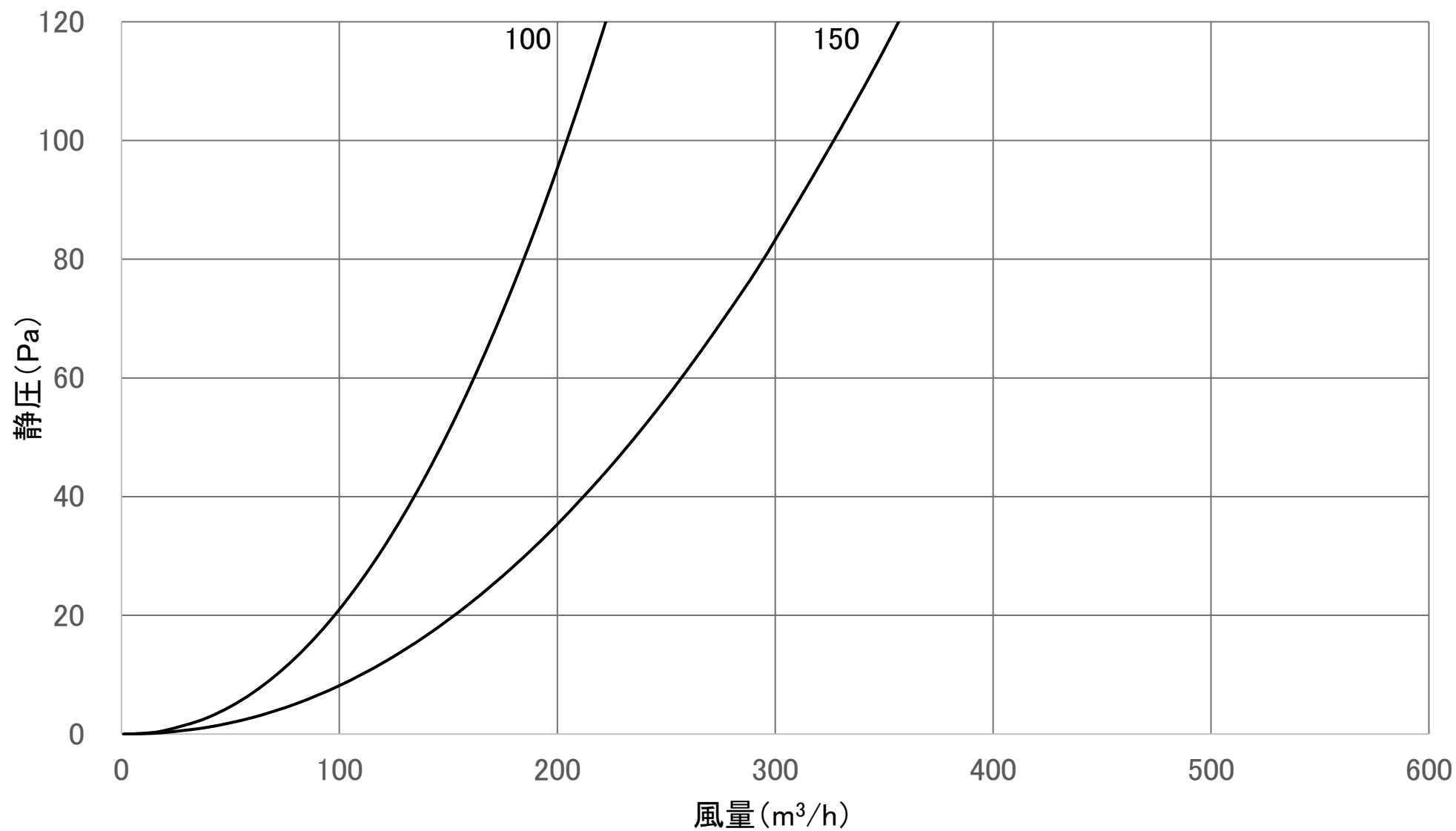
風量特性曲線 NTK(排気)
