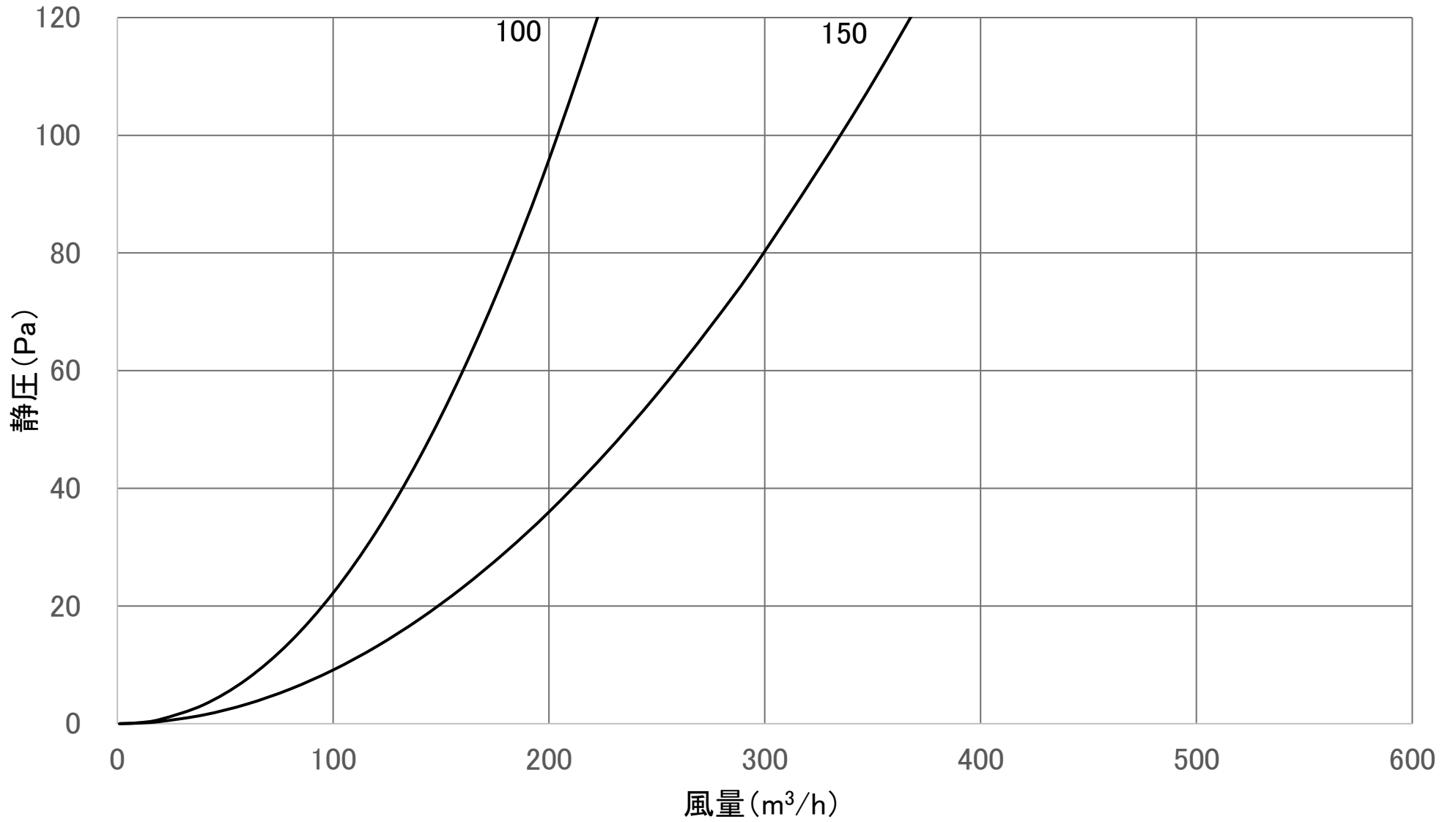
風量特性曲線 MAP2(排氣)
