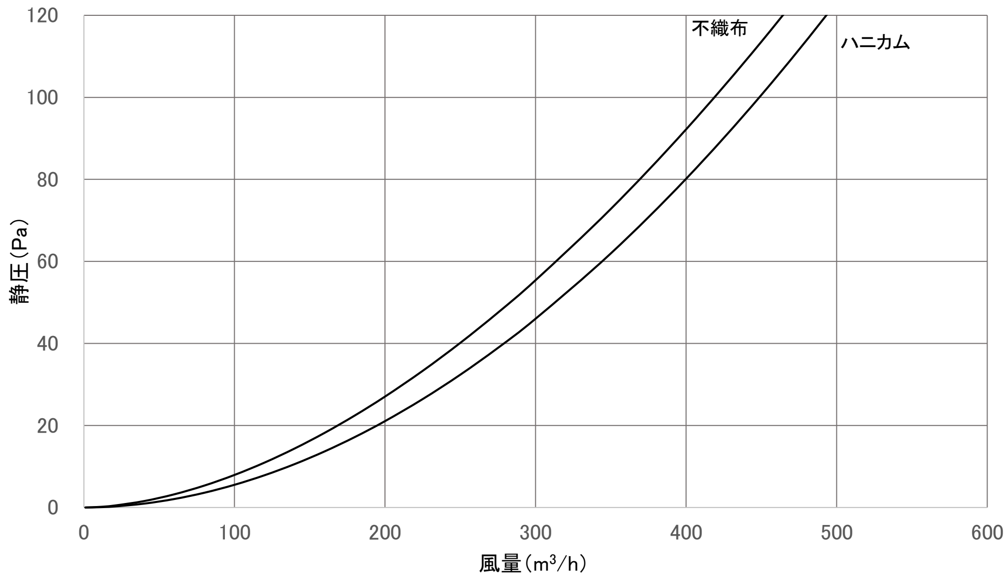
風量特性曲線 EQSI2-150
