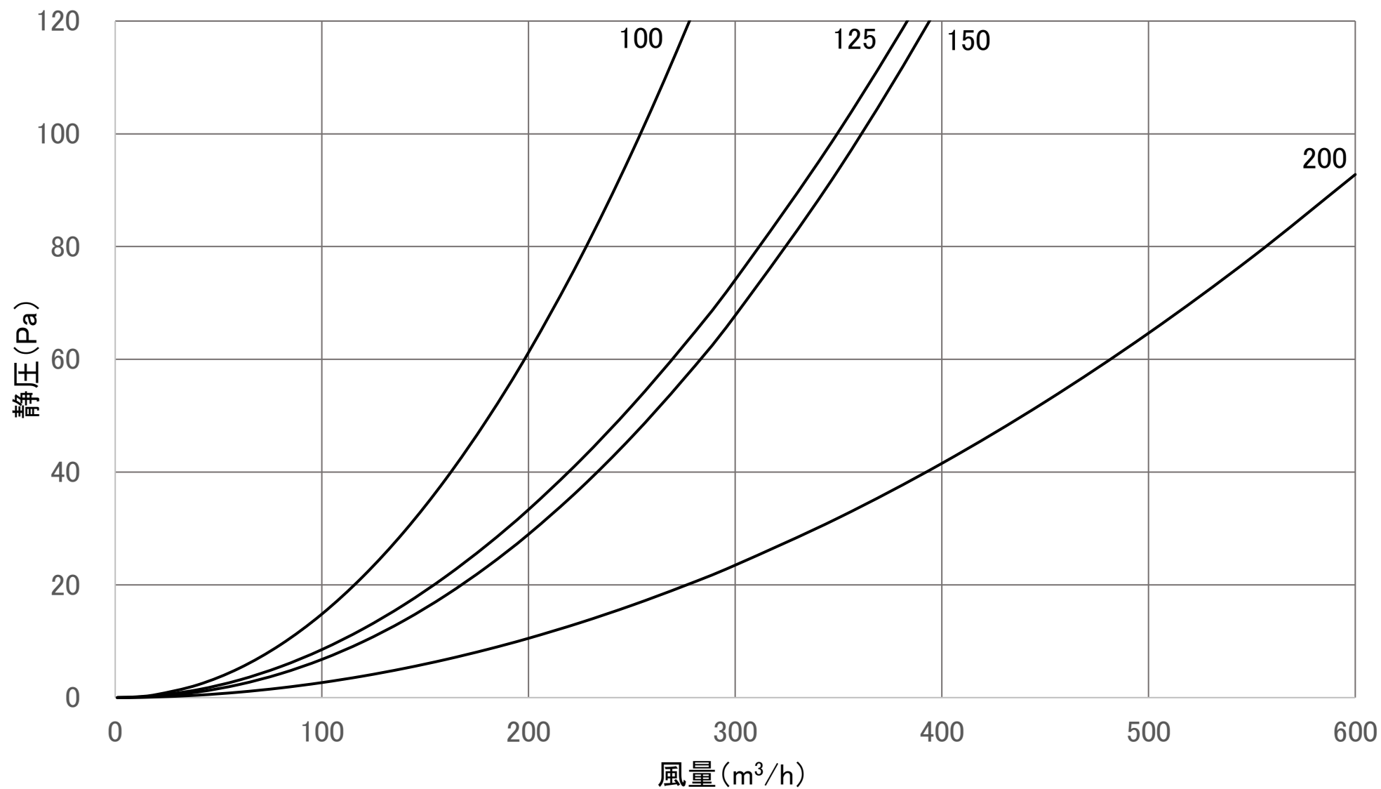
風量特性曲線 CRSG(排気)
