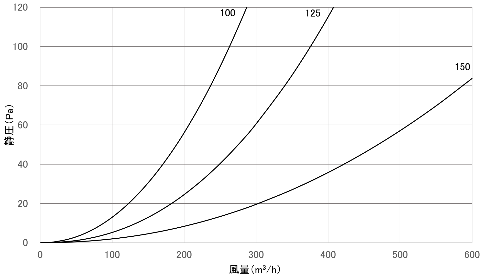
風量特性曲線 3LP(排氣)
