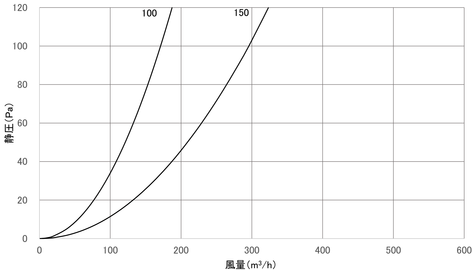
風量特性曲線 CRSBG(排気)
