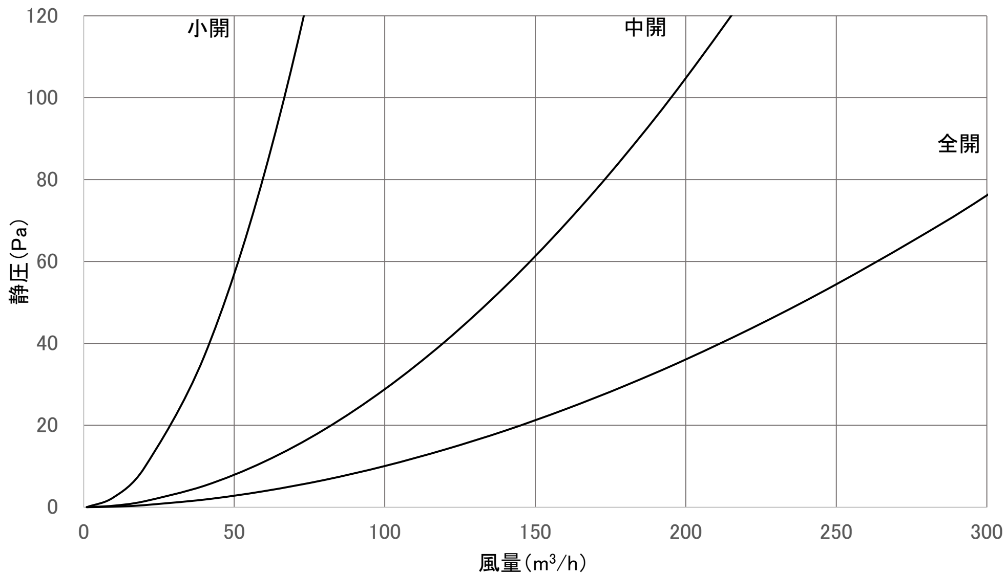
風量特性曲線 QSSC2-100(吸気)
