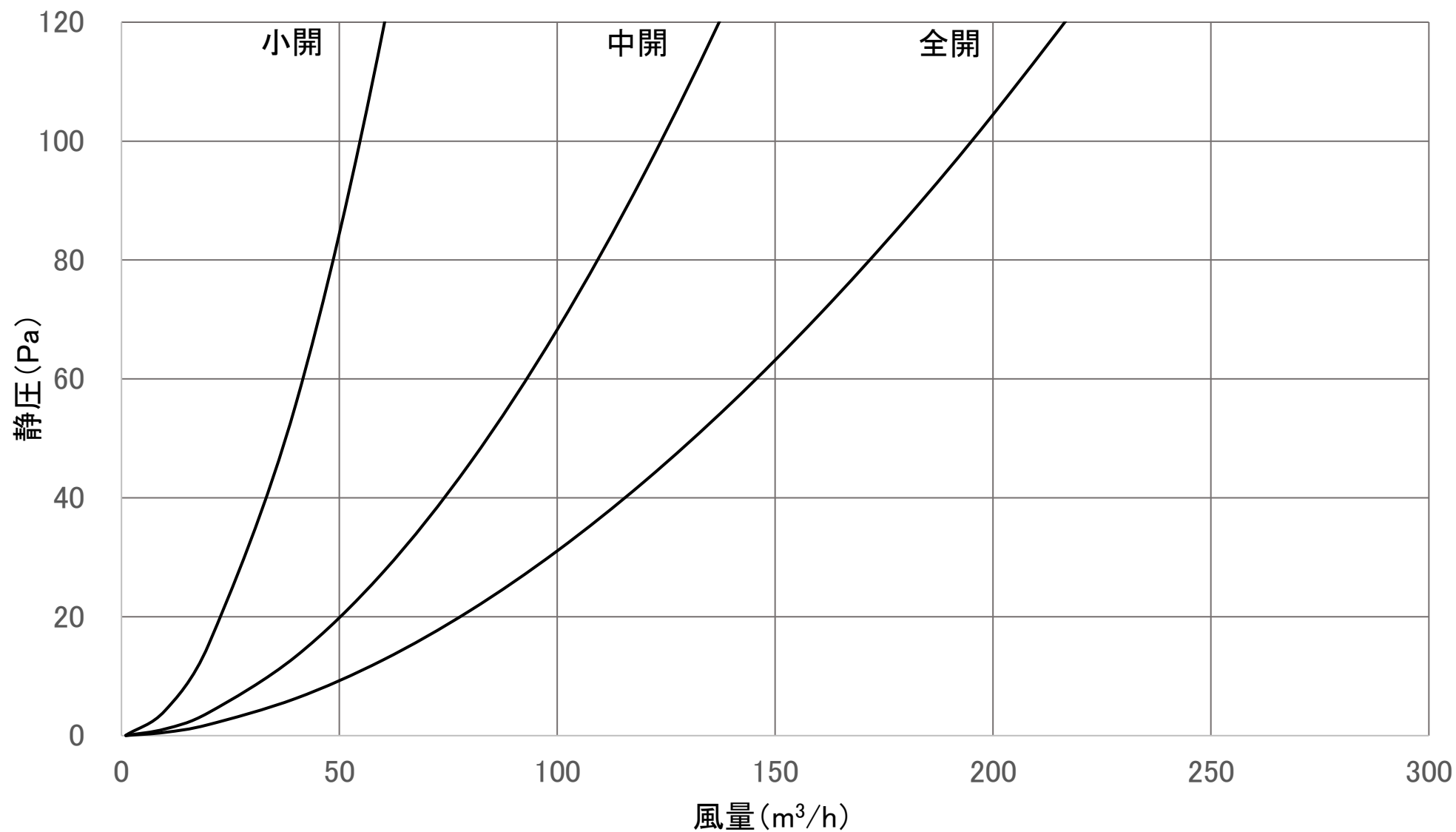
風量特性曲線 QSSC2-100H(吸気)
