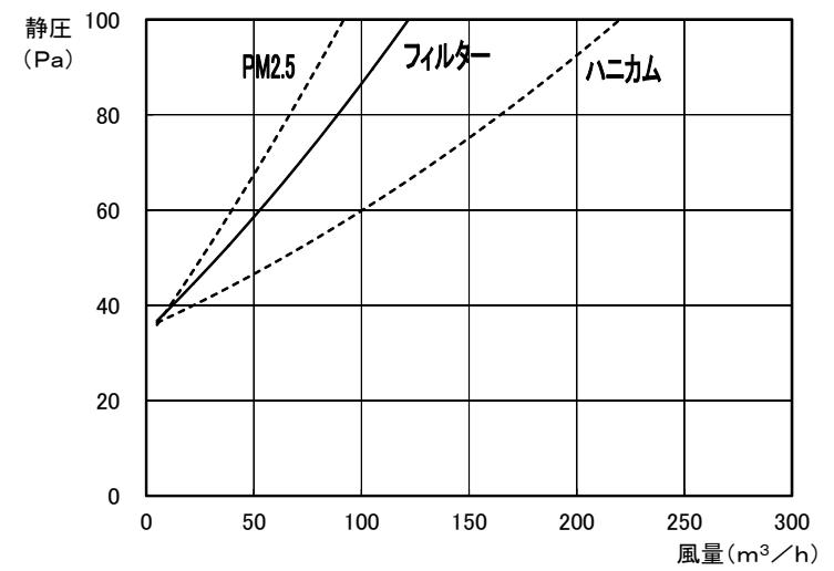
圧力損失曲線 *PM2.5フィルター・ハニカムフィルターはオプション
