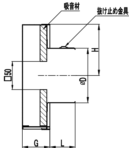
A-A 断面図
