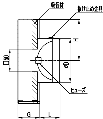
A-A 断面図
