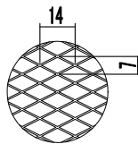
ワシヨシ ラシ網 7×14 (呼称・5メッシュ)
