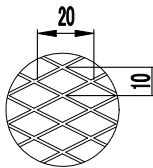
ラシ網 10×20 (呼称・3メッシュ)
