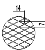
ワシヨシ ラシ網 7×14 (呼称・5メッシュ)
