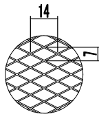
オプションメッシュ網 7×14 (呼称・5メッシュ)
