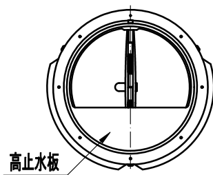
背面図(1:2)
