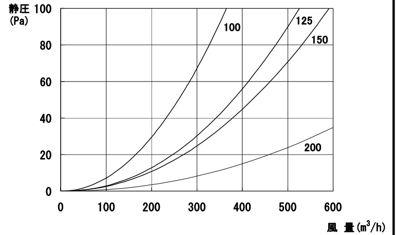
圧力損失曲線
