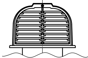
ガラリ詳細図(1:2)
