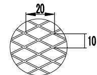
ラス網 10×20 (呼称・3メッシュ)
