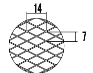
オプション ラス網 7×14 (呼称・5メッシュ)
