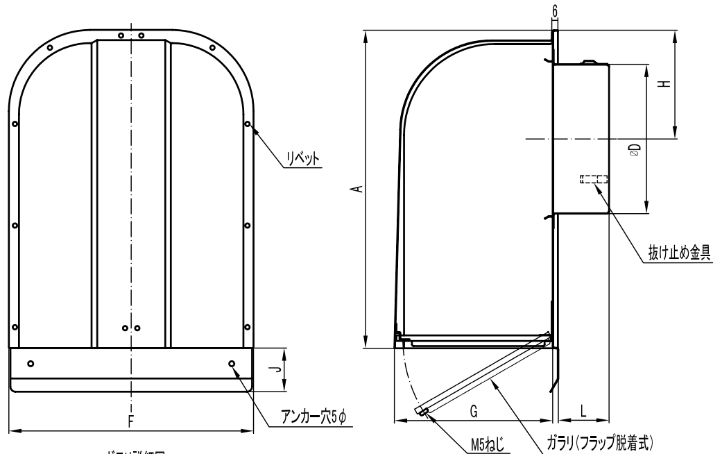
ガラー詳細図
