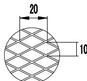
ワズ網 10×20 (呼称・3メッシュ)
