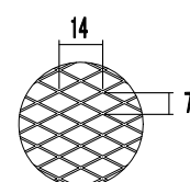
オプション ワズ網 7×14 (呼称・5メッシュ)
