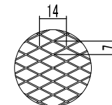
オプション ラス網 7×14 (呼称・5メッシュ)
