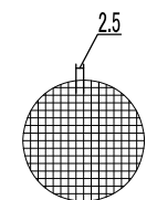
平織網 2.5×2.5 (呼称・10メッシュ)
