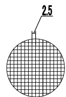
平織網 2.5×2.5 (呼称・10メッシュ)
