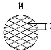
ワジョン ヲメ網 7×14 (呼称・5メッシュ)
