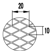
ヲメ網 10×20 (呼称・3メッシュ)
