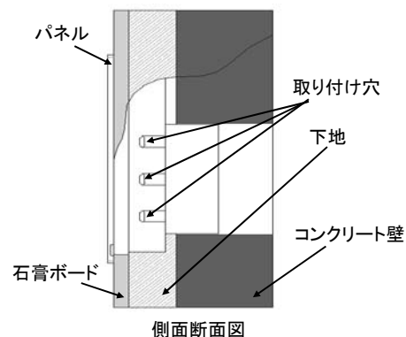
側面断面図
