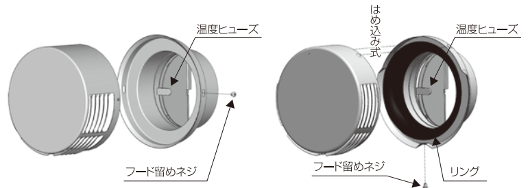
ダンパー部分拡大図
