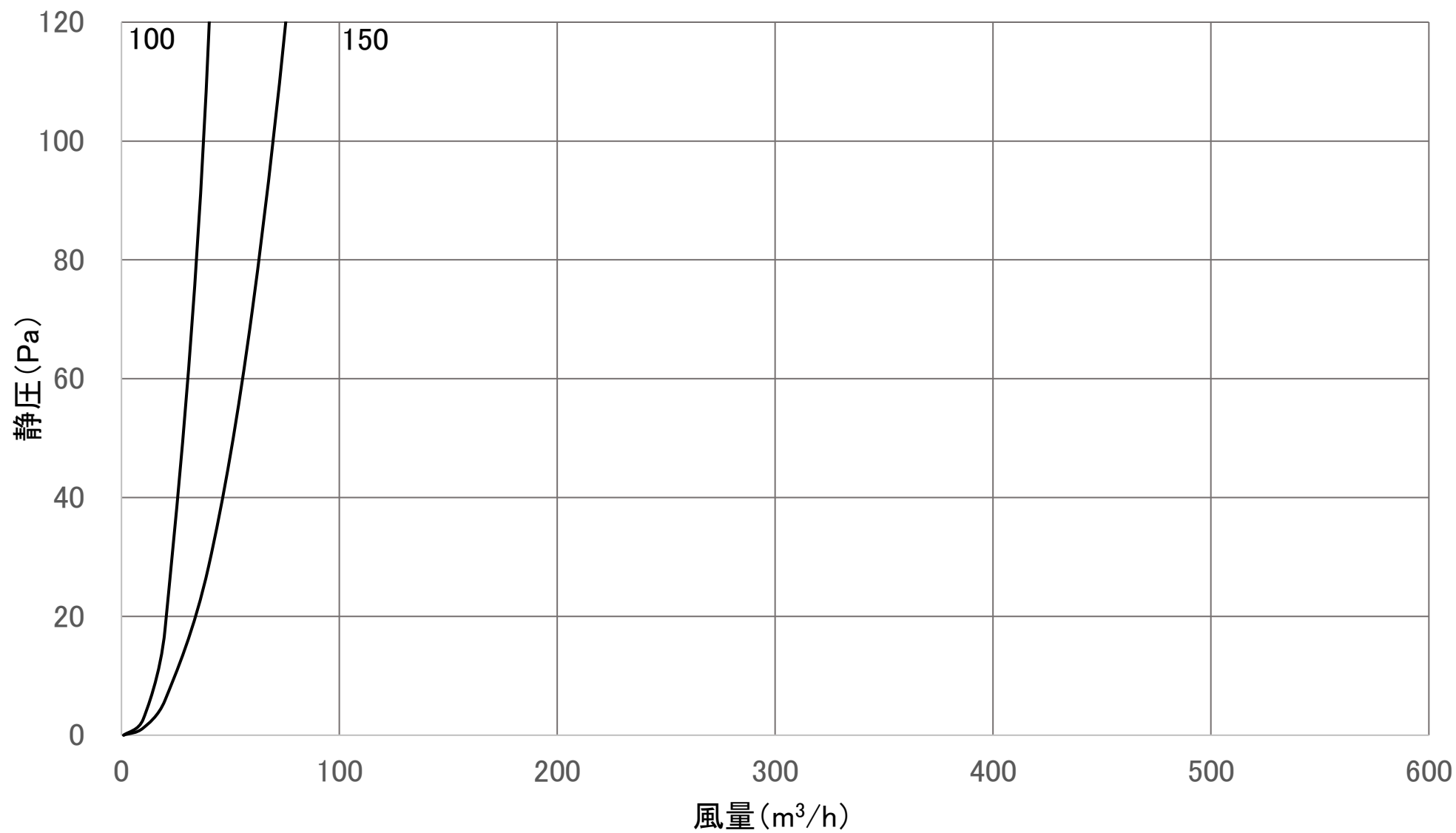
風量特性曲線 BSF-10M(吸気)
