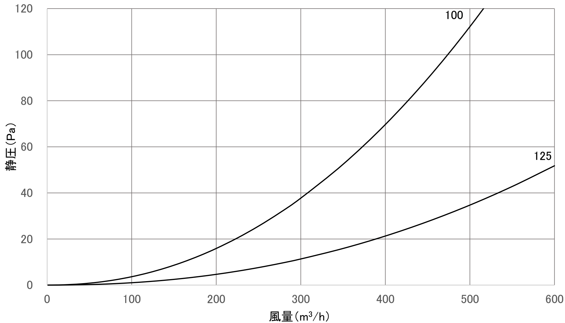
風量特性曲線 3KP(排気)
